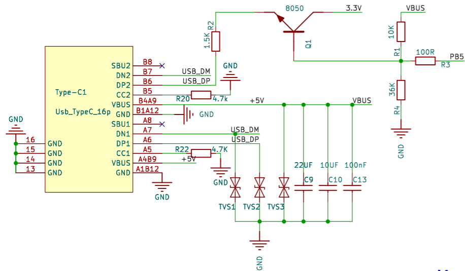
Type-C接口
